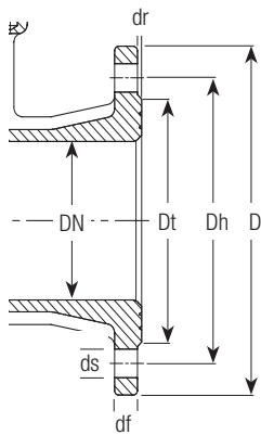
Drillings to ISO 7005 part 2 (EN 1092-2: 1997, DIN 2501):
